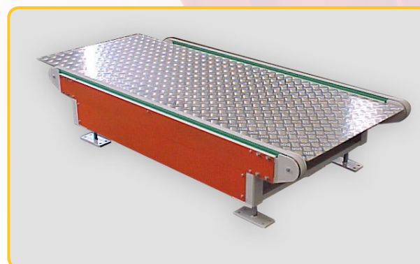
Trasportatore a doppia cinghia per trasporto elettrodomestici di medie dimensioni.
